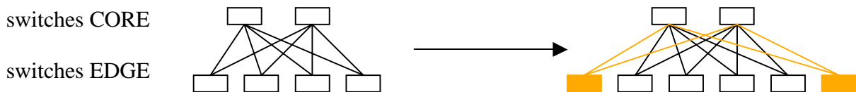
Figure 11 - Exemple d'évolution d'une architecture core-edge dual core
